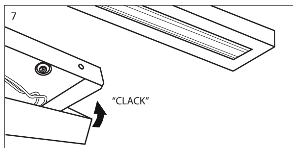
KIT DI SOSPENSIONE PER FIG. 1-2-3 SOSPENSION KIT FOR FIG. 1-2-3
