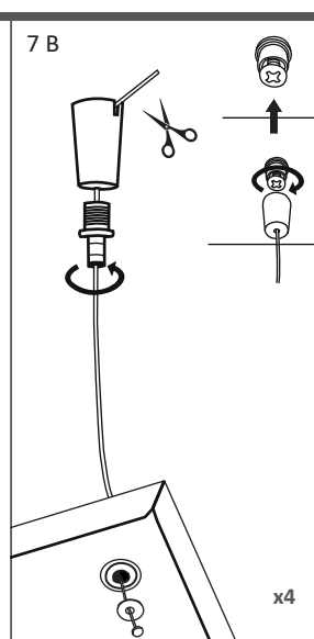
KIT DI SOSPENSIONE PER FIG. 4-5-6 SOSPENSION KIT FOR FIG. 4-5-6
